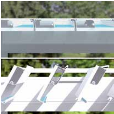
Evacuation d'eau contrôlée même en cas d'ouverture des lames
