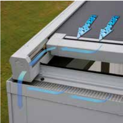
Evacuation d'eau intégrée
