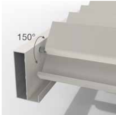
Orientable à 150°
