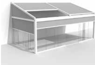
Lagune équipée de panneaux coulissants en verre et de Fixscreens intégrés du côté Side et Front
